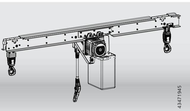
Doppelkettenzug KLDC-D: kurze Bauhöhe, Ablaufposition 2/4
